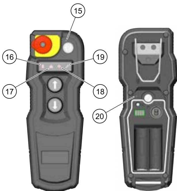
Figura 5. Indicadores LED y alertas del control remoto
