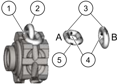
Figura 9. Áreas de desgaste de la cadena
