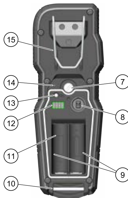
Figure 4. Dos de la télécommande
