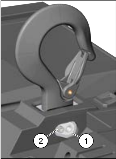
Figure 7. Retenue de la goupille de suspension/vis de retenue
