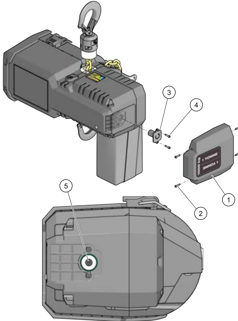
Figura 15. Procedimiento de descenso manual
