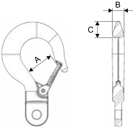
Figure 8. Critères d'enlèvement des crochets
