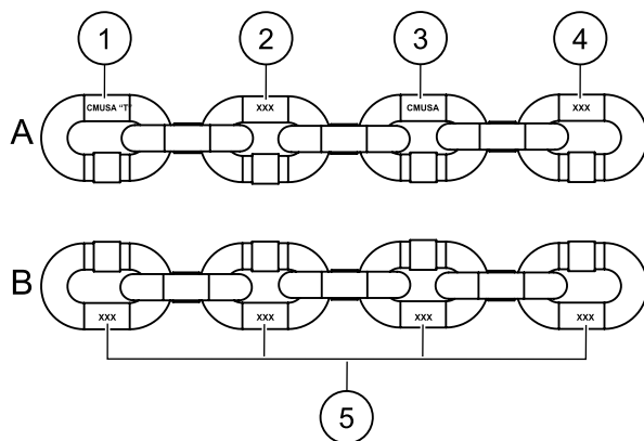
Figura 12. Relieves de la cadena
