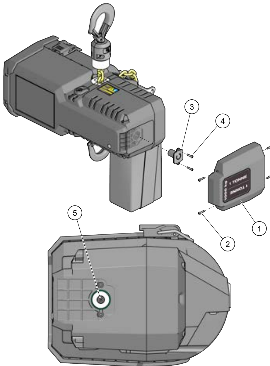
Figura 15. Procedimento de descida manual
